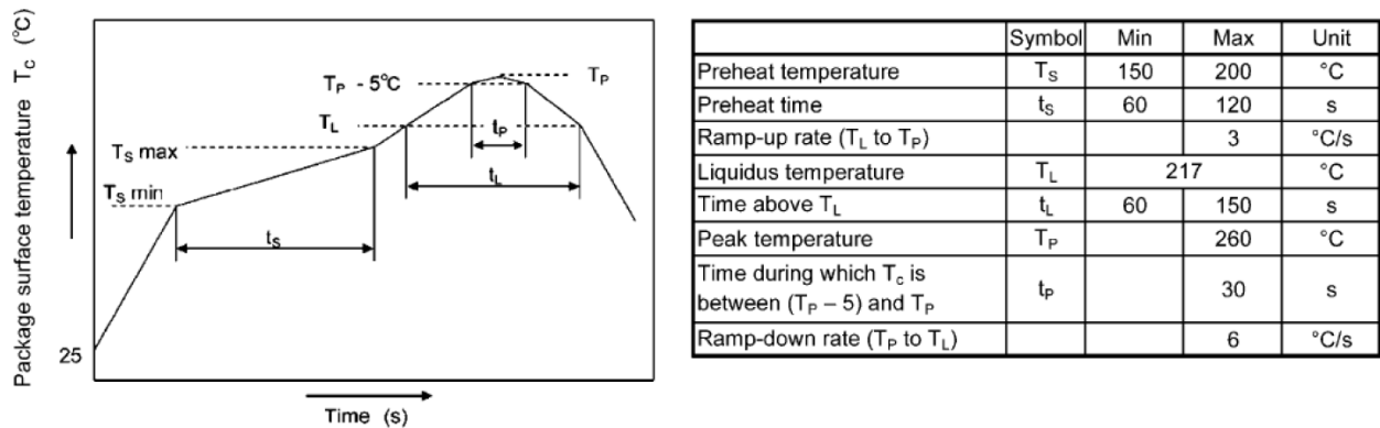
图 8 回流焊参数
