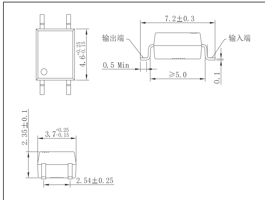
图 4 HSSR-S1A08-2 外形尺寸
